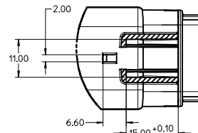
SECTION D-D
