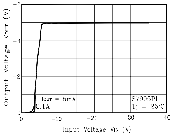
Fig. 1 V_{OUT} - V_{IN}
