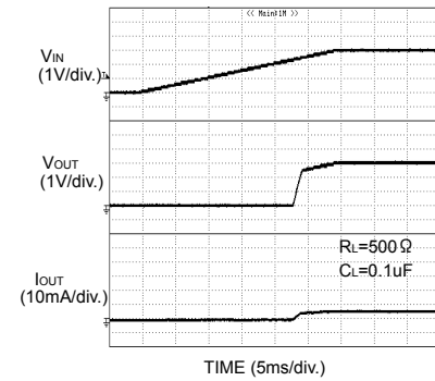
Fig.36 UVLO V_{IN} rising
