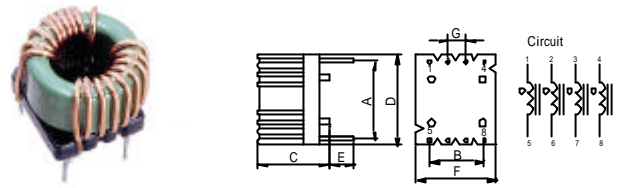
BCB1104RI-330-N
