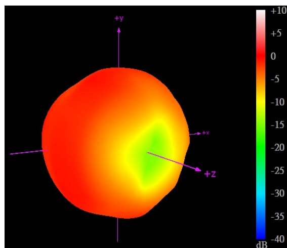
2500MHz
