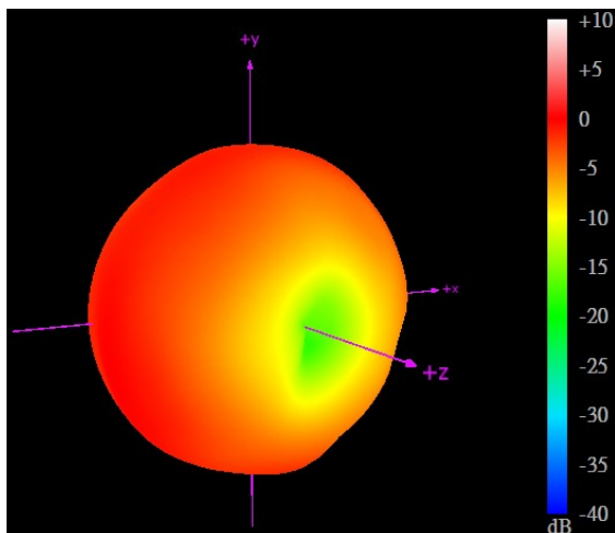
2400MHz
