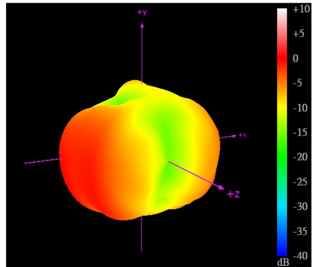
2540MHz
