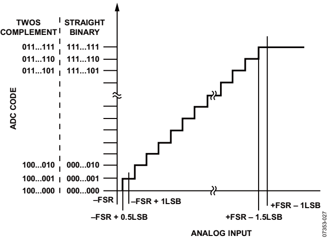
图25. ADC理想传递函数
