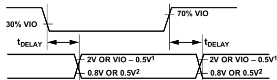
图3.时序的电平
