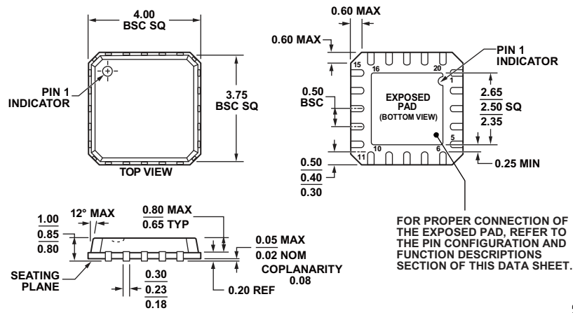
图44. 20引脚LFCSP_VQ封装, 4 mm x 4 mm四方超薄体 (CP-20-4), 尺寸单位: mm
