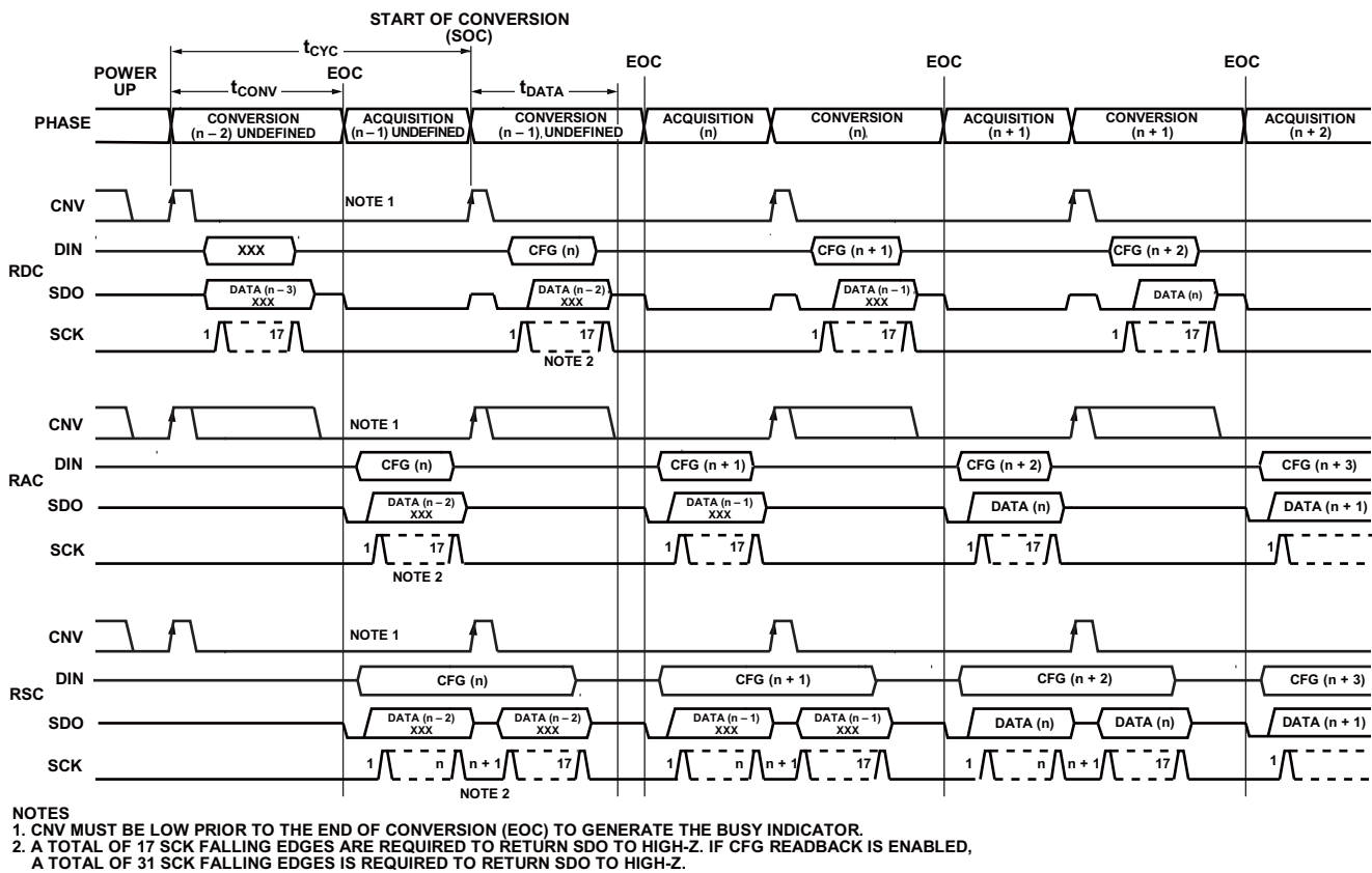
图38. 含繁忙指示器的AD7682/AD7689通用接口时序
