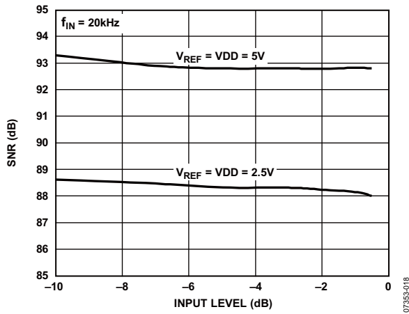
图19. SNR与输入电平的关系
