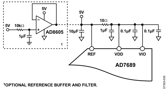
图36. 应用电路示例
