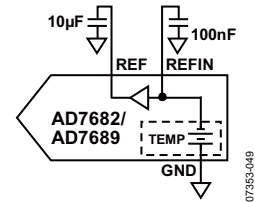
图31. 2.5 V或4.096 V内部基准电压源连接
