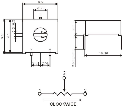
TSR-3386G
