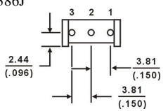
TSR-3386S
