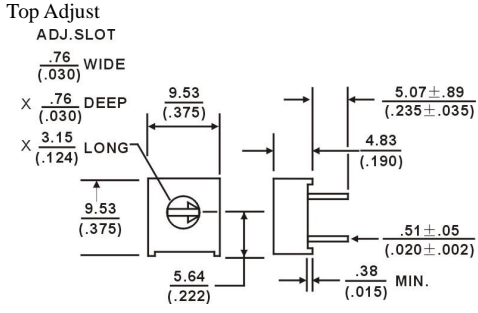
TSR-3386F
