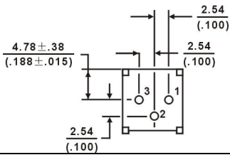
TSR-3386R
