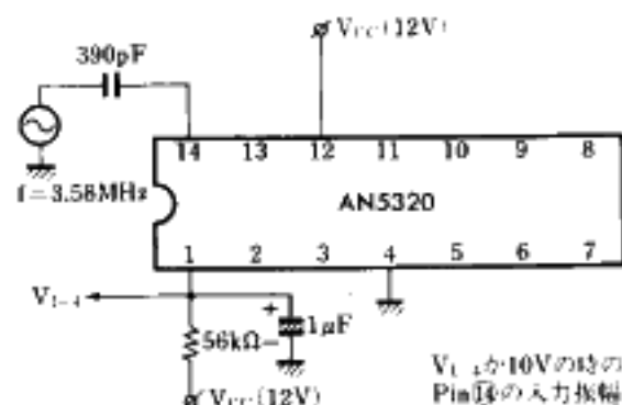
Test Circuit 2 (V SWN )
