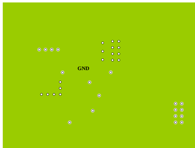
Inner2 Layer
