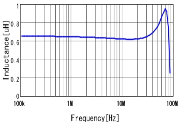
■DFE201610P-R68M L
