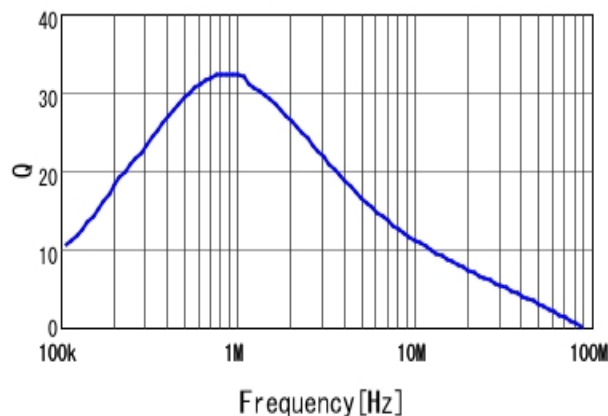
■DFE201610P-R68M Q
