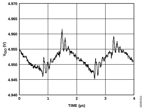
图11. V_{ISO} = 5\text{ V} 输出电压典型纹波，90%负载
