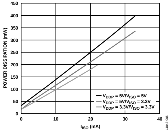
图5. 典型总功耗与 I_{ISO} 的关系
