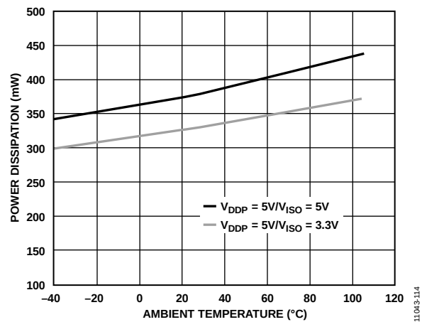
图14. 30 mA负载时功耗与温度的关系
