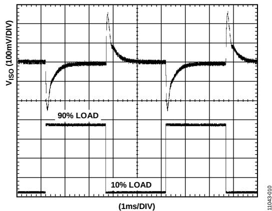
图10. 典型瞬态负载响应，5 V输入，3.3 V输出，10%至90%负载阶跃
