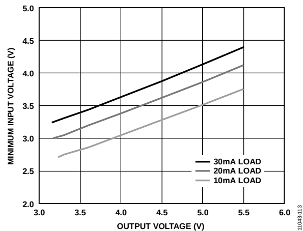
图13. 输出电压和所需输入电压之间的关系，负载未满载，保持PWM中占空系数大于80%
