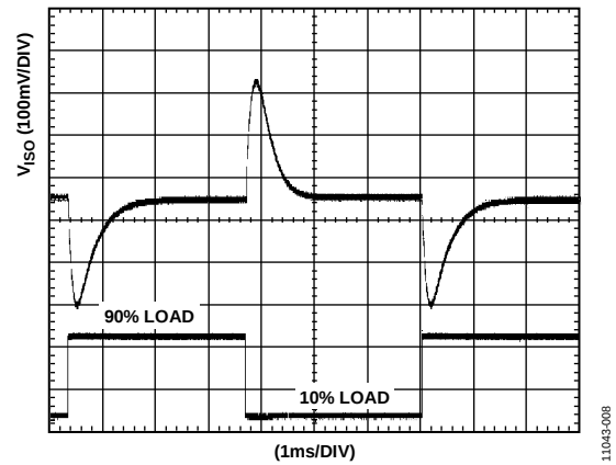
图8. 典型 V_{ISO} 瞬态负载响应, 5 V输入, 5 V输出, 10%至90%负载阶跃
