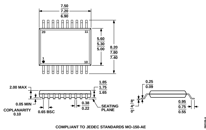
图22. 20引脚紧缩小型封装[SSOP] (RS-20)
