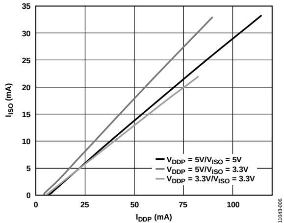
图6. 5 V/5 V、5 V/3.3 V和3.3 V/3.3 V时典型隔离输出电源电流 I_{ISO} 与外部负载的关系
