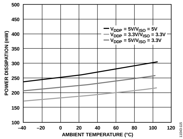
图15. 20 mA负载时功耗与温度的关系
