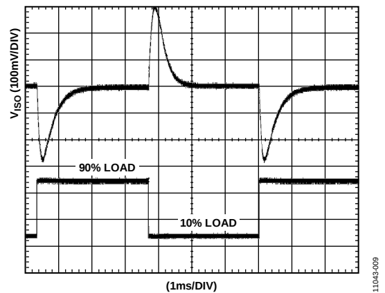
图9. 典型瞬态负载响应, 3.3 V输入, 3.3 V输出, 10%至90%负载阶跃
