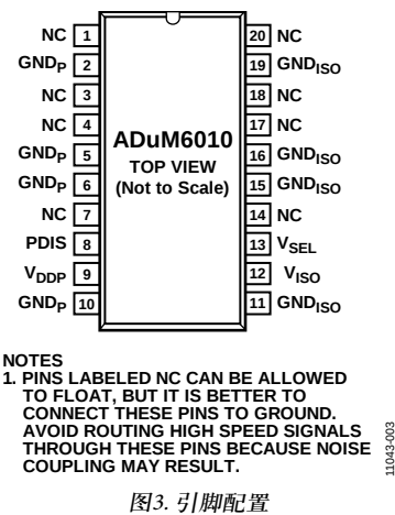
图3. 引脚配置
