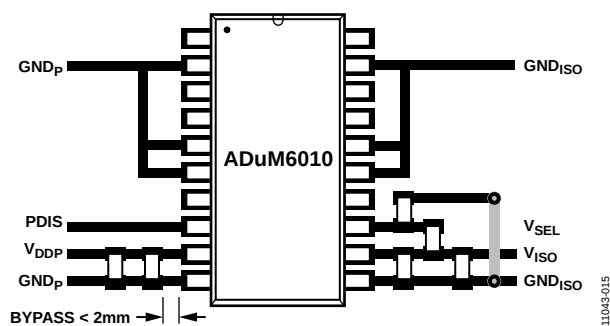
图18. 推荐的PCB布局
