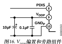
图16. V_{DDP} 偏置和旁路组件
