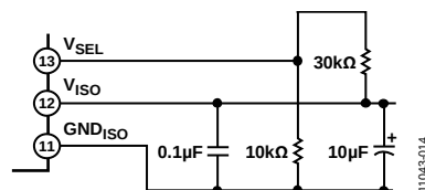
图17. V_{ISO} 偏置和旁路组件
