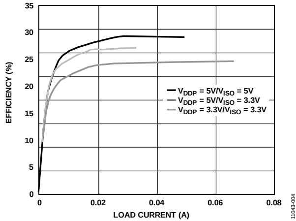
图4. 5 V/5 V、5 V/3.3 V和3.3 V/3.3 V的典型电源效率
