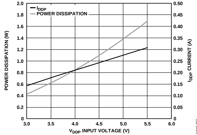
图7. 典型短路输入电流和功耗与 V_{DDP} 电源电压的关系
