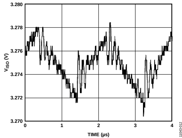
图12. V_{ISO} = 3.3\text{ V} 输出电压典型纹波，90%负载
