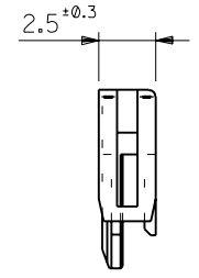
断面 E-E SECT. E-E (8極以上) (OVER 8CKT.)
