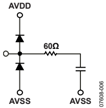
Figure 11. CCDIN (Pin 22)
