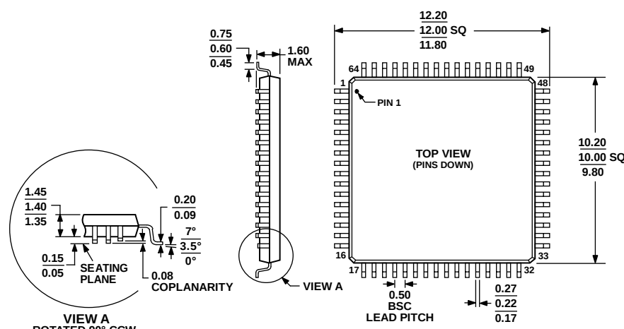
图10. 64引脚薄型四方扁平封装[LQFP] (ST-64-2) 尺寸单位: mm
