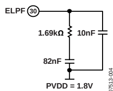
图8. ELPF元件
