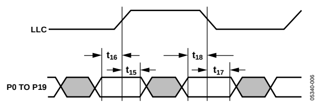
图5. 像素端口和控制DDR输出时序(CP内核)
