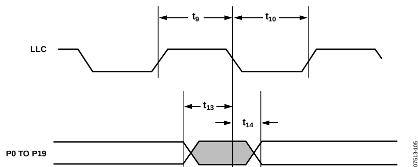
图4. 像素端口和控制SDR输出时序(CP内核)
