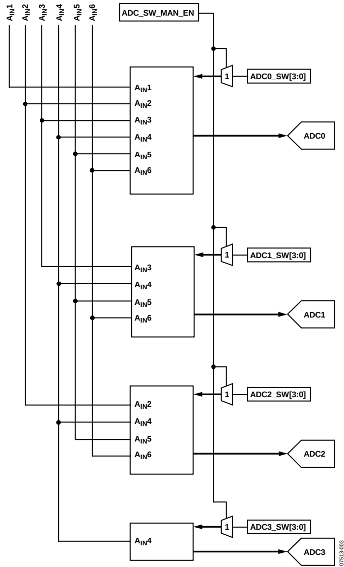
图7. 内部引脚连接
