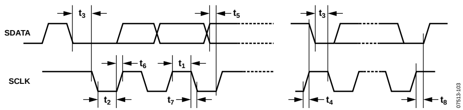
图2. I²C时序
