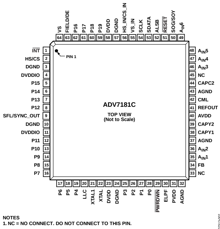
图6. 引脚配置
