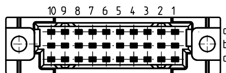
bestückt / assemble
