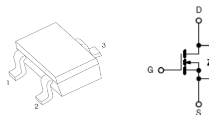
SOT - 523
