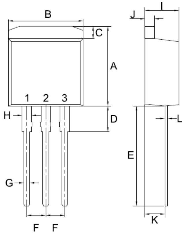
TO-262 (I 2 PAK)
