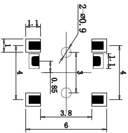
PCB板位置尺寸
