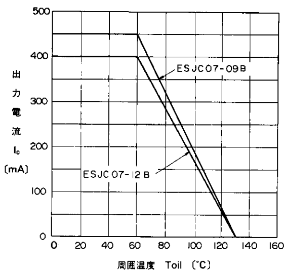
電流低減特性曲線 Current Derating Curve
