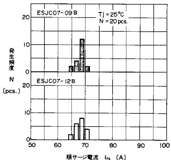
順サージ電流耐量特性分布 (代表特性) Forward Surge Current
