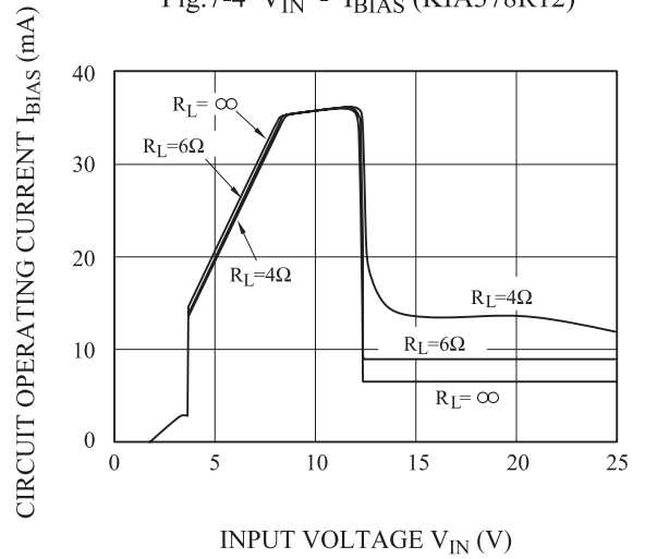
Fig.7-4 V_{IN} - I_{BIAS} (KIA378R12)
