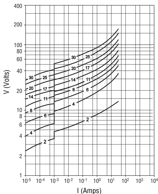
Model Size 0603 - (ZV 2 M 0603 300 HT ~ ZV 30 K 0603 300 HT)
