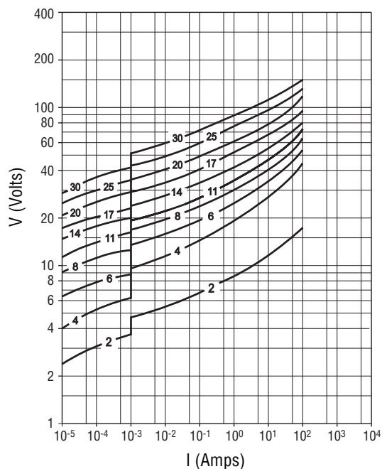
Model Size 0805 - (ZV 2 M 0805 xxx HT ~ ZV 30 K 0805 xxx HT)
