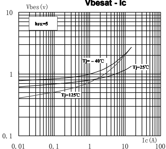
V_{besat} - I_c
