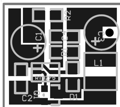
- Top Layer -
