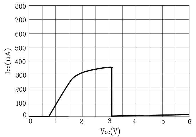
Fig. 2 I_{CC} - V_{CC}
