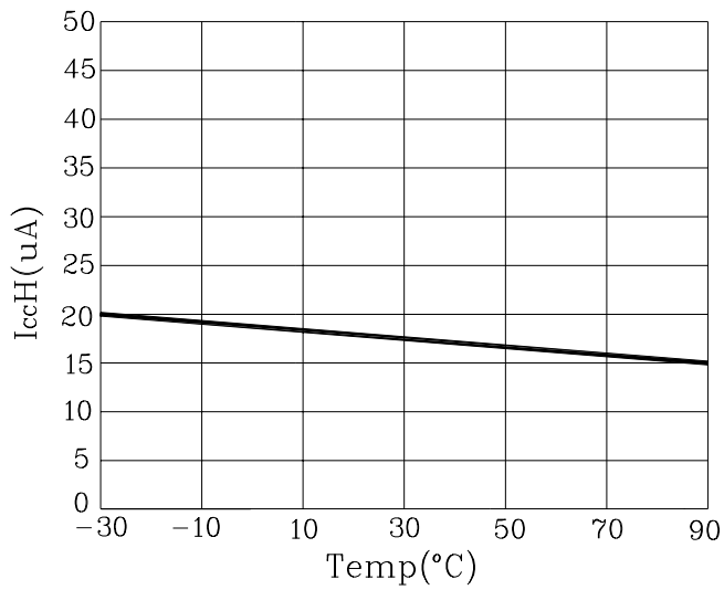
Fig. 3 I_{CCH} - \text{Temp}
