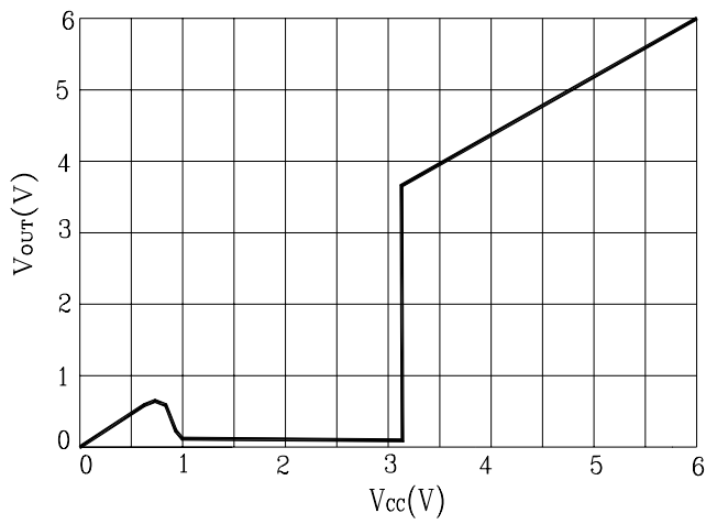
Fig. 1 V_{OUT} - V_{CC}
