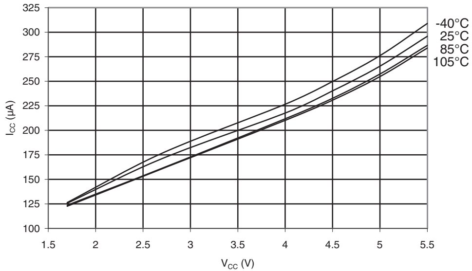
Figure 34-41. ATmega168PA: ADC Current vs. V CC (AREF = AV CC )
