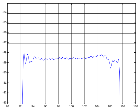
Phase Linearity( f_0 \pm 6.75\text{MHz} )
