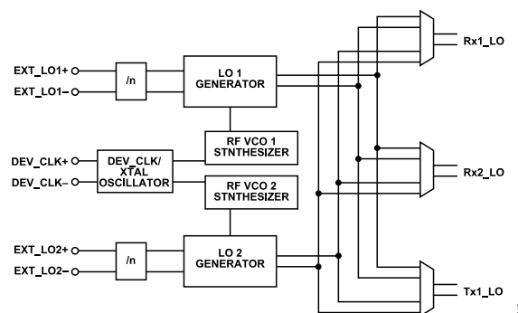
Figure 12. RF LO
