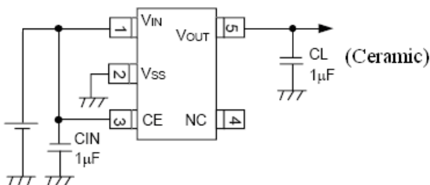
LR6218E (SOT23-5)
