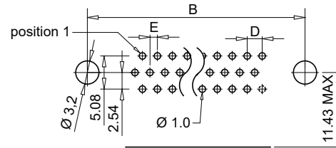
EDGE OF P.C.BOARD
