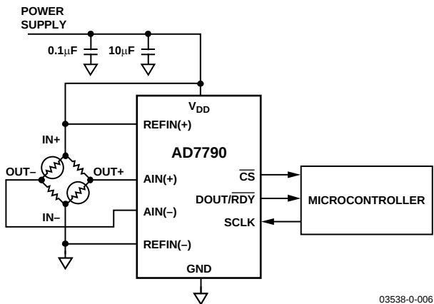
图7. 基本连接图
