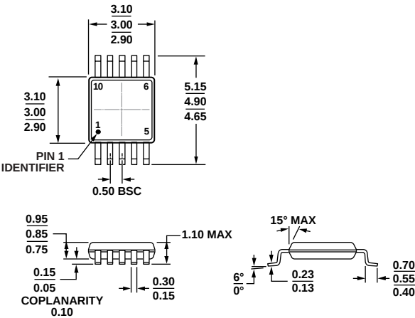
COMPLIANT TO JEDEC STANDARDS MO-187-BA 图11. 10引脚超小型封装[MSOP] (RM-10) 图示尺寸单位: mm
