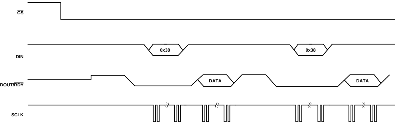
图9. 连续转换
