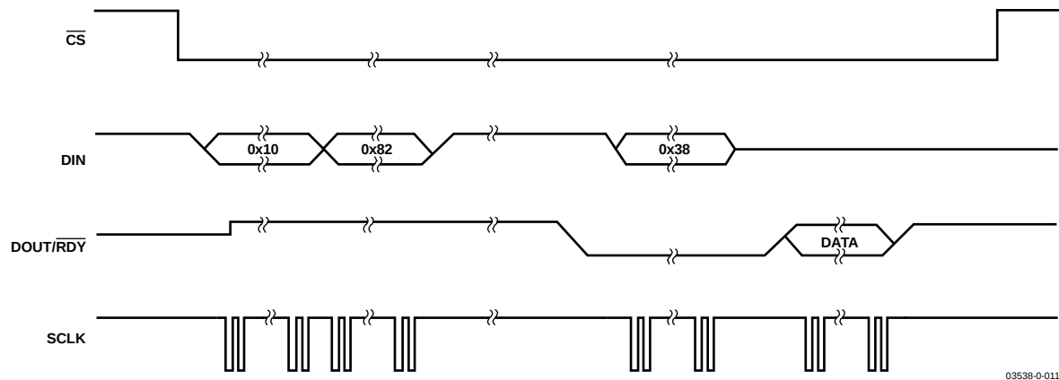
图8. 单次转换
