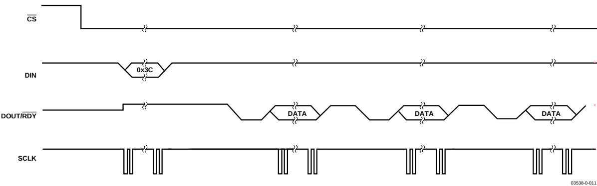
图10. 连续读取
