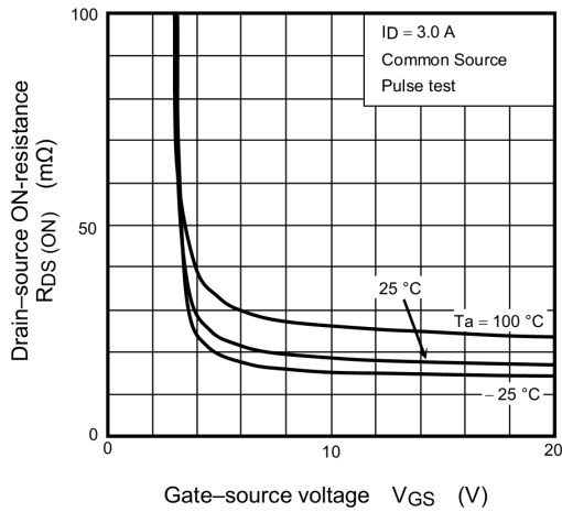
Fig. 7.3 R_{DS(ON)} - V_{GS}
