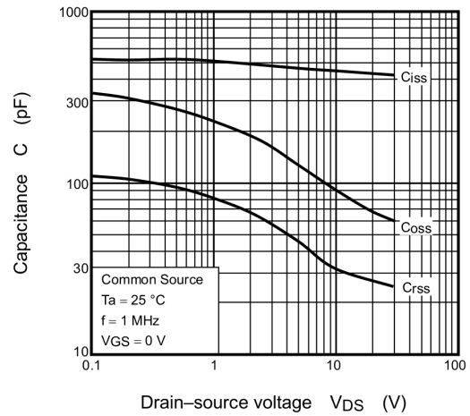
Fig. 7.8 C - V_{DS}
