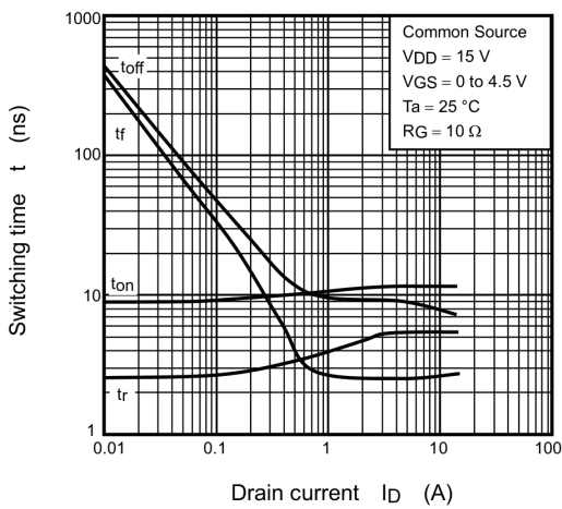
Fig. 7.9 t - I_D
