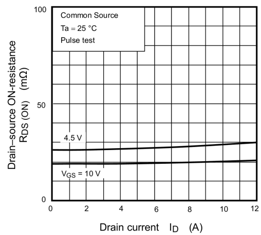
Fig. 7.4 R_{DS(ON)} - I_D
