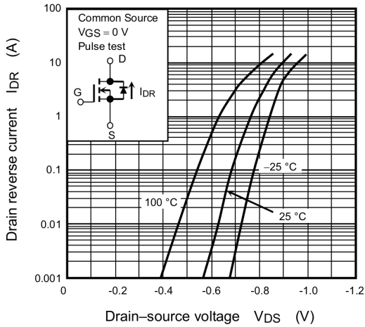
Fig. 7.7 I_{DR} - V_{DS}
