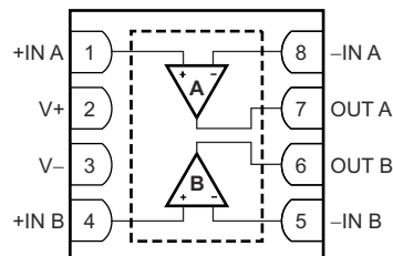
图 6-2. DRG (WSO-8) Package, Top View
