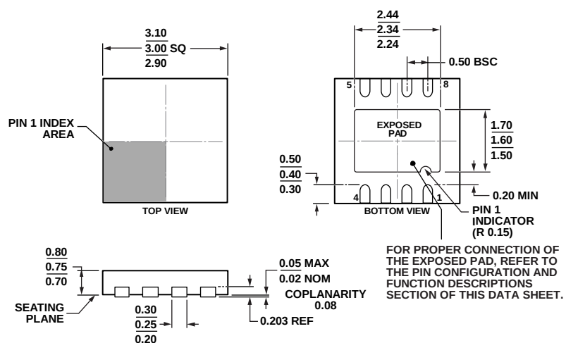
图71. 8引脚脚架构芯片级封装[LFCSP_WD]
