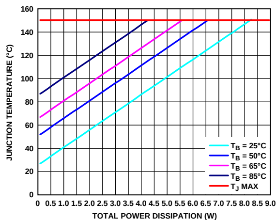
图67. 8引脚LFCSP的结温与总功耗的关系
