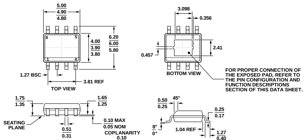
图72. 8引脚标准小型封装, 带裸露焊盘[SOIC_N_EP]
