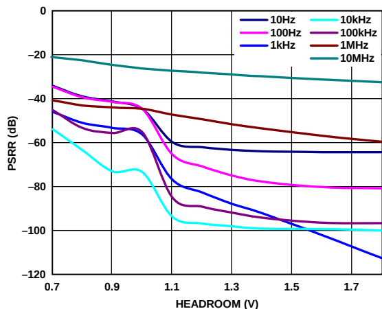
图30. 电源抑制比(PSRR)与裕量电压的关系, ADM7151-04, V_{IN} = 5\text{ V} , 800 mA负载
