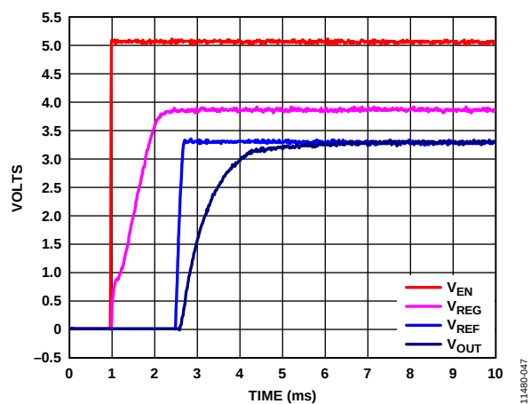
图47. V_{IN} 上升后的 V_{OUT} 、 V_{REF} 、 V_{REG} 启动时间, V_{OUT} = 3.3\text{ V} , V_{IN} = 5\text{ V}
