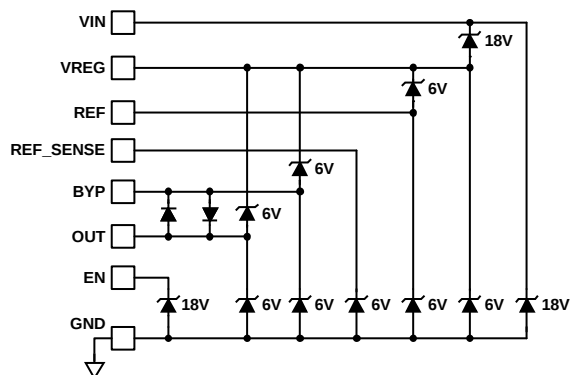
图50. 简化ESD保护功能框图
