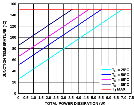
图68. 8引脚SOIC的结温与总功耗的关系
