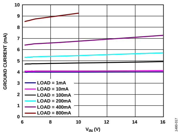
图17. 接地电流与输入电压( V_{IN} )的关系, ADM7151-04, V_{OUT} = 5V
