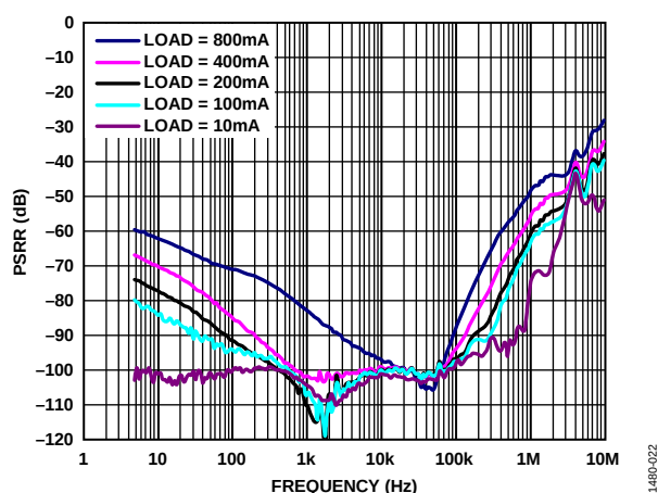
图22. 电源抑制比(PSRR)与频率的关系, ADM7151-04, V_{IN} = 5V
