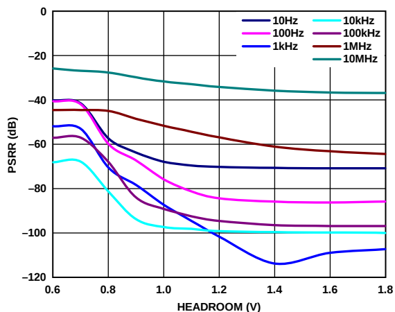
图29. 电源抑制比(PSRR)与裕量电压的关系, ADM7151-04, V_{IN} = 5\text{ V} , 400 mA负载
