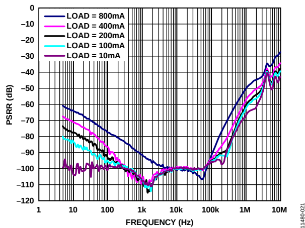
图21. 电源抑制比(PSRR)与频率的关系, ADM7151-02, V_{IN} = 4V
