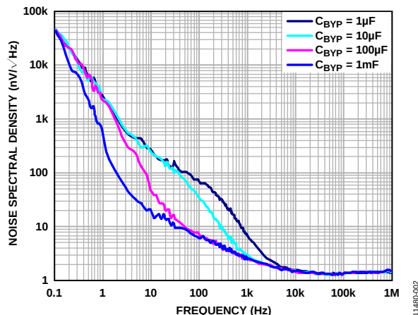
图2. 不同CBYP下噪声频谱密度(NSD)与频率的关系
