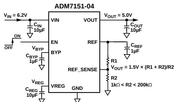
图49. 典型可调输出电压应用原理图
