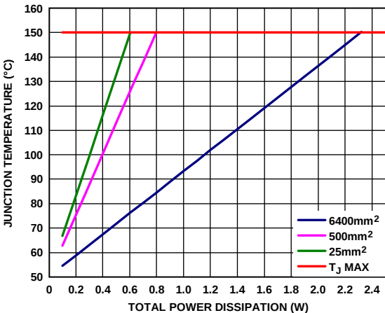
图62. 8引脚LFCSP的结温与总功耗的关系， T_A = 50^\circ\text{C}
