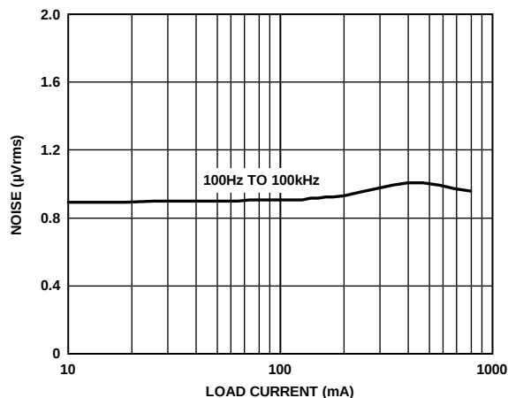
图32. RMS输出噪声与负载电流( I_{LOAD} )的关系, 100 Hz至100 kHz, ADM7151-04, V_{OUT} = 5\text{ V}
