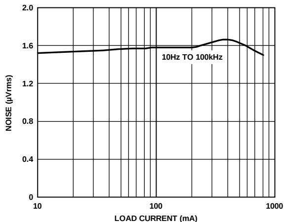
图31. RMS输出噪声与负载电流( I_{LOAD} )的关系, 10 Hz至100 kHz, ADM7151-04, V_{OUT} = 5\text{ V}
