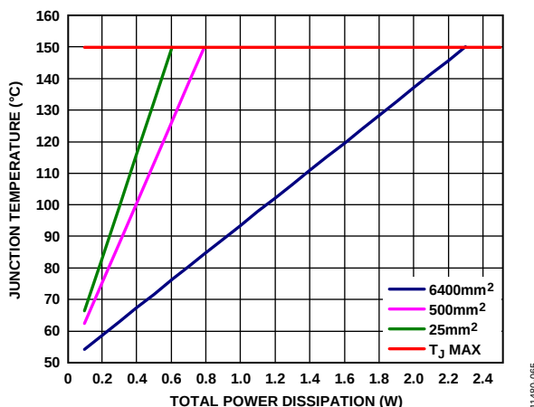
图65. 8引脚SOIC的结温与总功耗的关系, T_A = 50^\circ\text{C}
