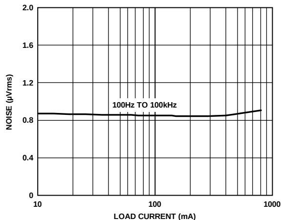
图34. RMS输出噪声与负载电流( I_{LOAD} )的关系, 100 Hz至100 kHz, ADM7151-02, V_{OUT} = 4\text{ V}
