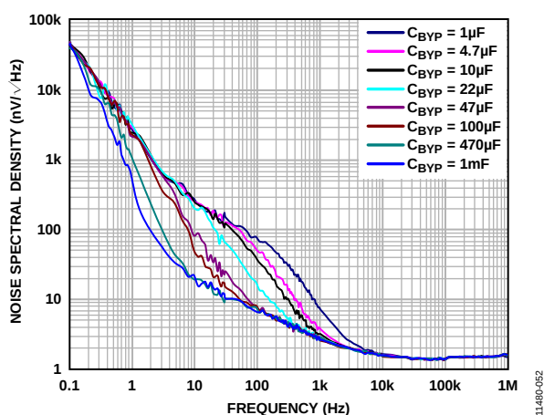
图52. 噪声频谱密度与频率的关系， C_{\text{BYP}} = 1 \mu\text{F} 至 1 mF
