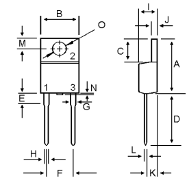
TO-220A
