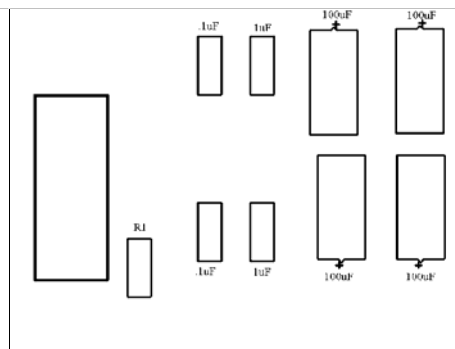
Fig. 2b. Layer 1 silkscreen
