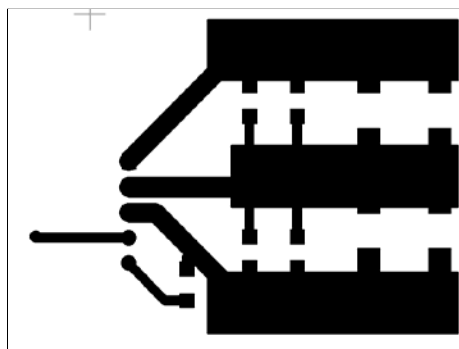
Fig. 2a. Layer 1 conductor.
