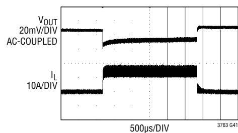
15A Load Step
