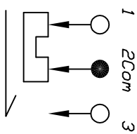
CIRCUIT: SPDT
