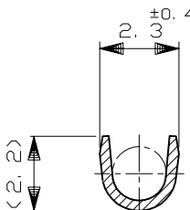
断面 A-A SECT A-A ( 175026のみ適用 ) ( ONLY 175026 )
