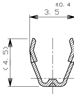
断面 B-B SECT B-B ( 175026のみ適用 ) ( ONLY 175026 )
