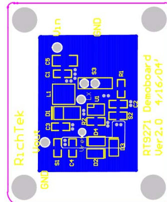
- Bottom Layer -
