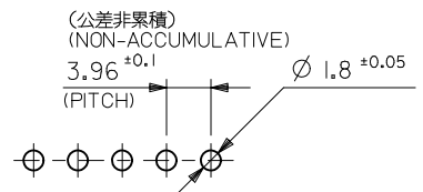
基板取付穴推奨寸法 RECOMMENDED P.C.BOARD HOLE DIM.
