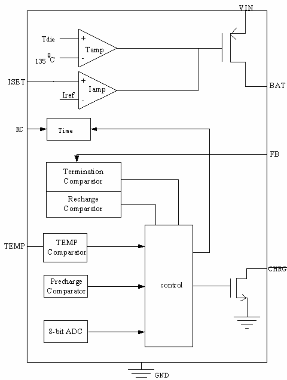
图 2 功能框图
