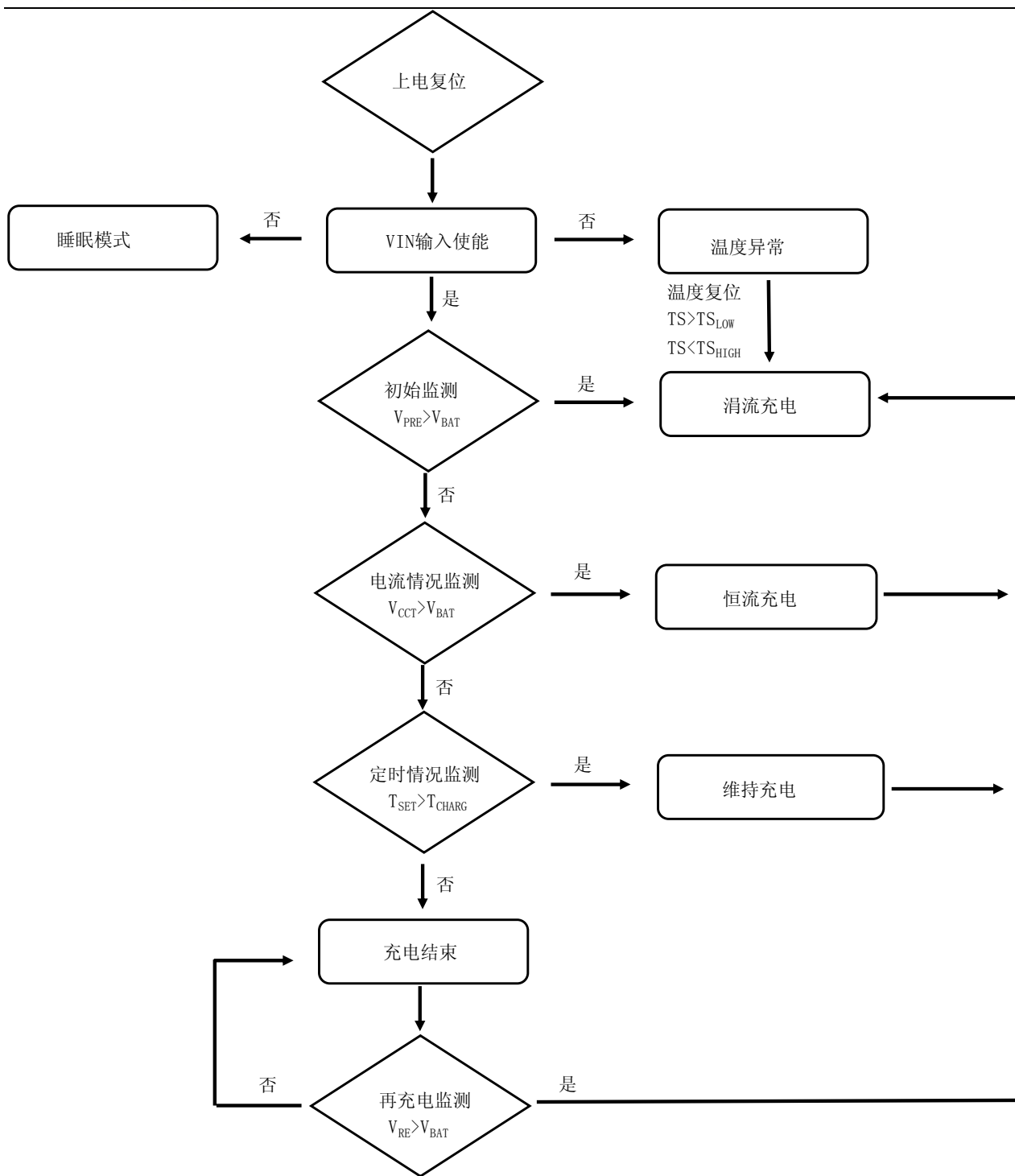
图4 充电工作框图
