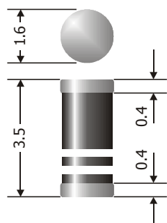
Dimensions - Maße [mm]
