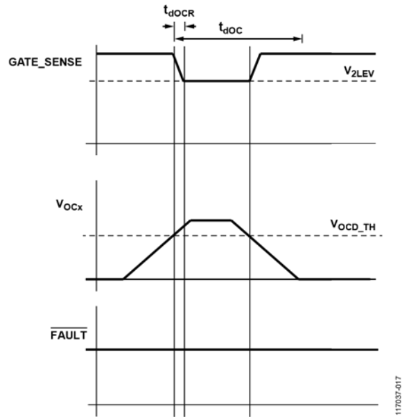
图17. 双电平定时器恢复示例
