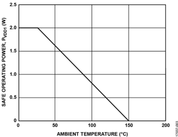
图3. 热减额曲线，依据DIN V VDE V 0884-10获得的安全限值与 ambient temperature 的关系
