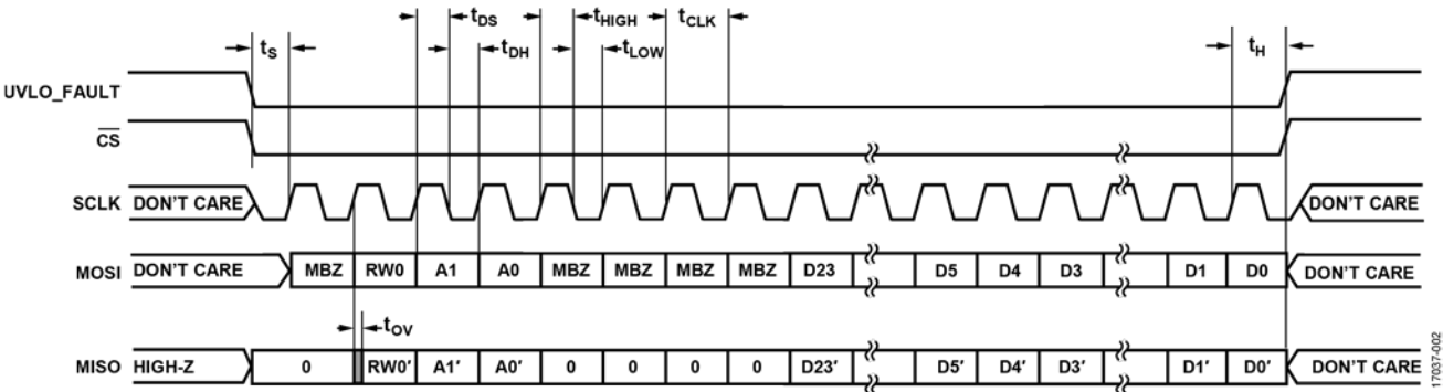
图2. SPI时序图
