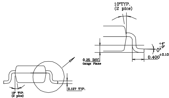
5-Pin TSOT-23 (D5)
