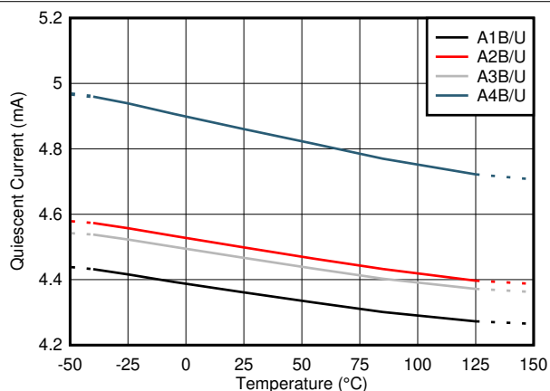
图 7-21. 静态电流与温度间的关系
