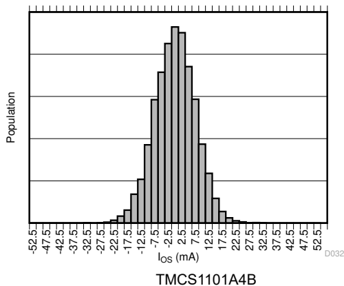
图 7-15. 输入失调电流产生分布
