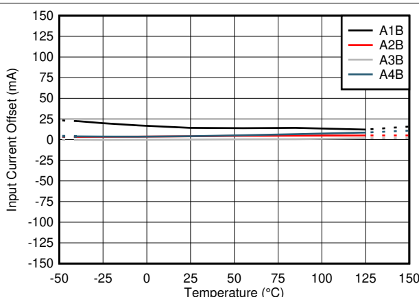
图 7-3. TMCS1101AxB 输入失调电流与温度间的关系
