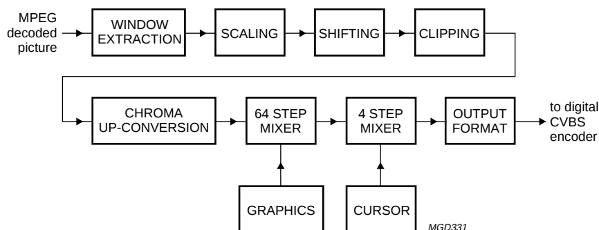
Fig.11 Display unit.
