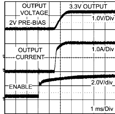
预偏置启动
