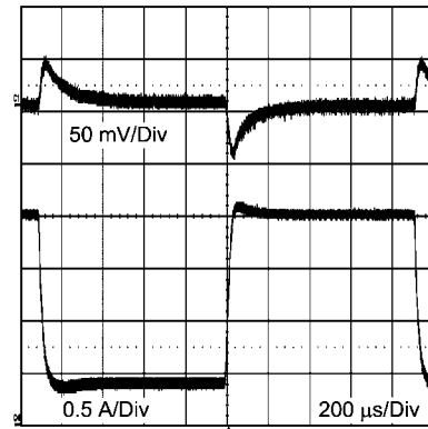
瞬态响应
