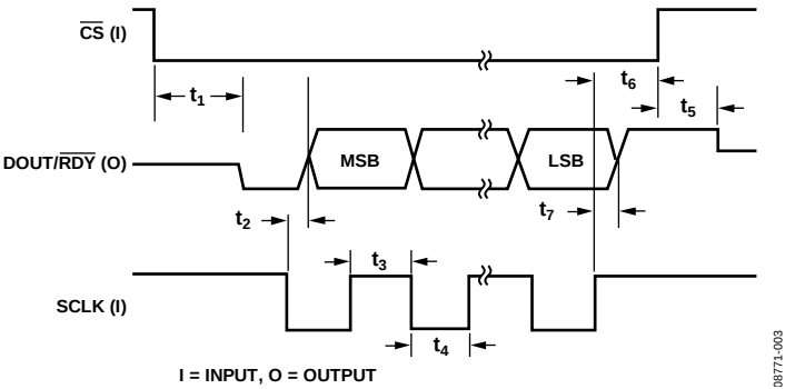
图3. 读取周期时序图
