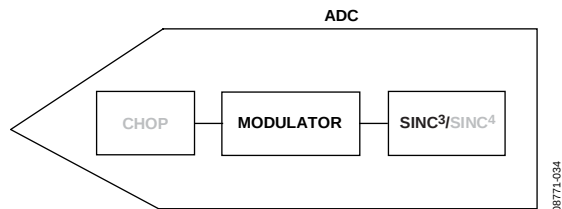
图32. \text{Sinc}^3 滤波器(斩波禁用)
