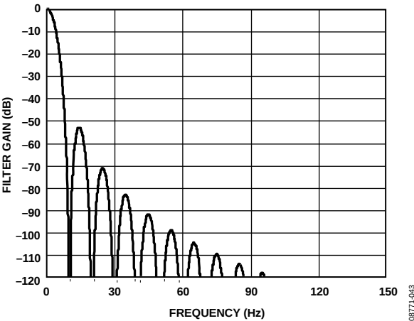
图30. Sinc 4 滤波器响应(FS[9:0] = 480)
