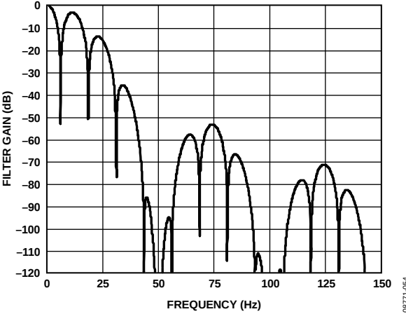
图43. Sinc 4 滤波器响应(FS[9:0] = 96，斩波使能)
