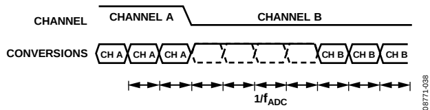
图25. Sinc 4 通道切换
