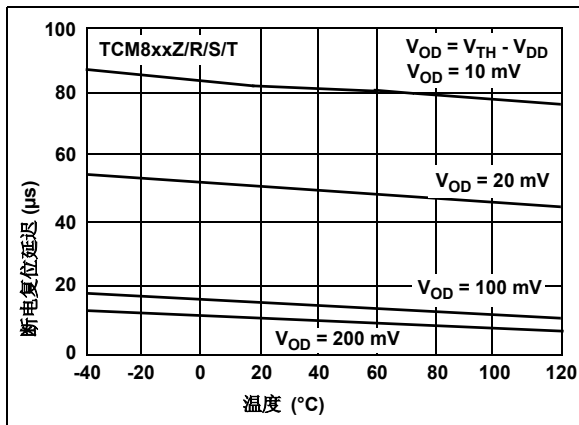
图 3-3: 断电复位延迟 - 温度曲线, SOT-23
