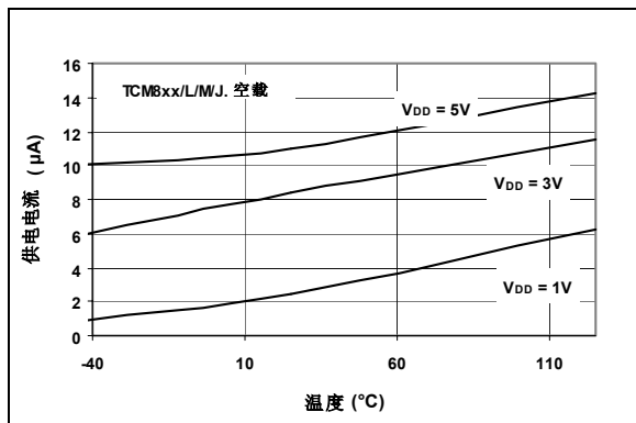
图 3-5: 供电电流 - 温度曲线, SC-70
