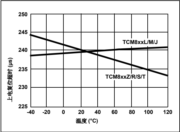
图 3-7: 上电复位超时 - 温度曲线, SOT-23
