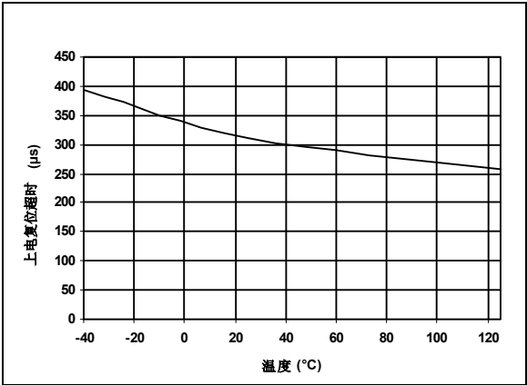
图 3-8: 上电复位超时 - 温度曲线, SC-70
