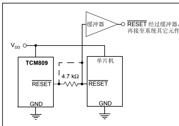
图 2-3: TCM809 至双向复位 I/O 的接口电路
