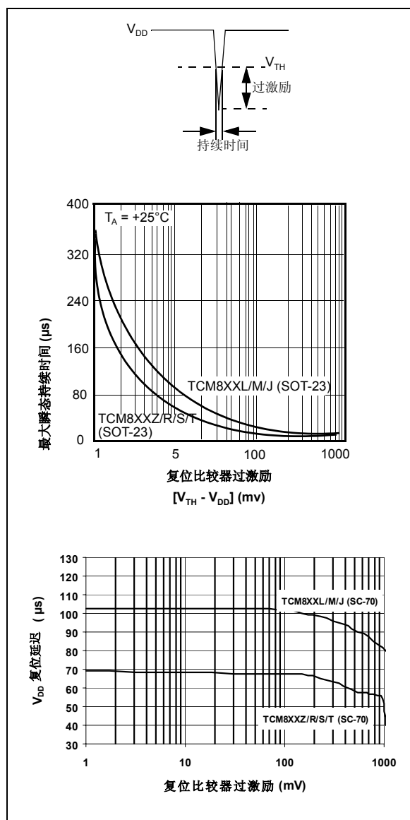
图 2-1: 器件可抑制的最大负向瞬态脉冲持续时间与最大负向瞬态脉冲幅度关系曲线 ( 25^{\circ}\text{C} )
