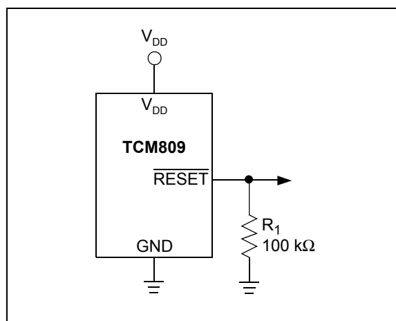
图 2-2: 在 TCM809 \overline{\text{RESET}} 输出引脚外接电阻 R_1 ，可确保在 V_{DD} = 0\text{V} 时 \overline{\text{RESET}} 输出有效。
