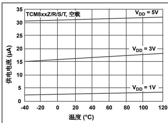
图 3-1: 供电电流 - 温度曲线, SOT-23
