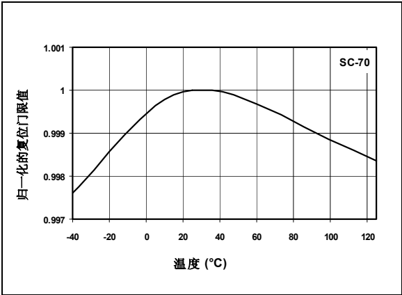
图 3-10: 归一化的复位门限值 - 温度曲线, SC-70
