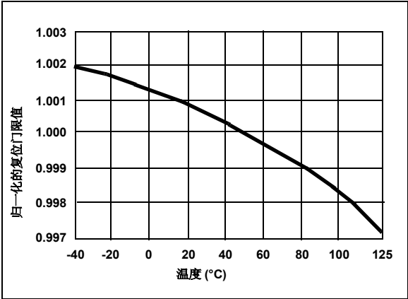
图 3-9: 归一化的复位门限值 - 温度曲线, SOT-23
