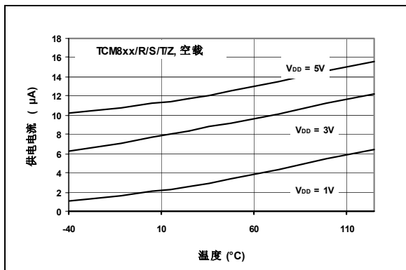
图 3-2: 供电电流 - 温度曲线, SC-70
