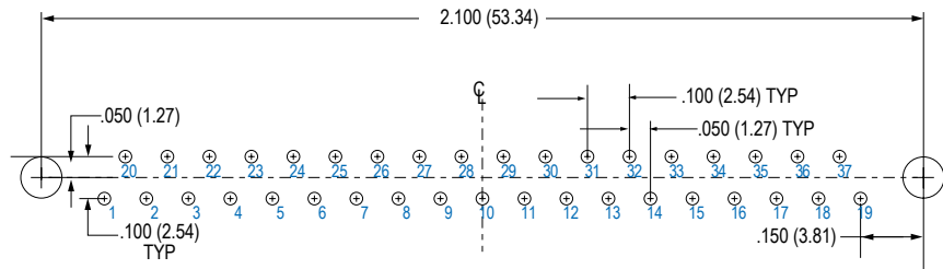
37 SOCKET MWDM-37SBS
